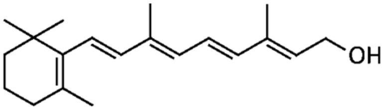
All-trans-retinol
