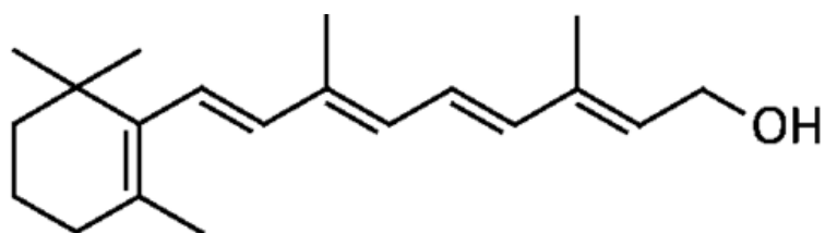
All-trans-retinol
