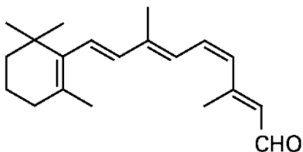
11-cis-Retinal
